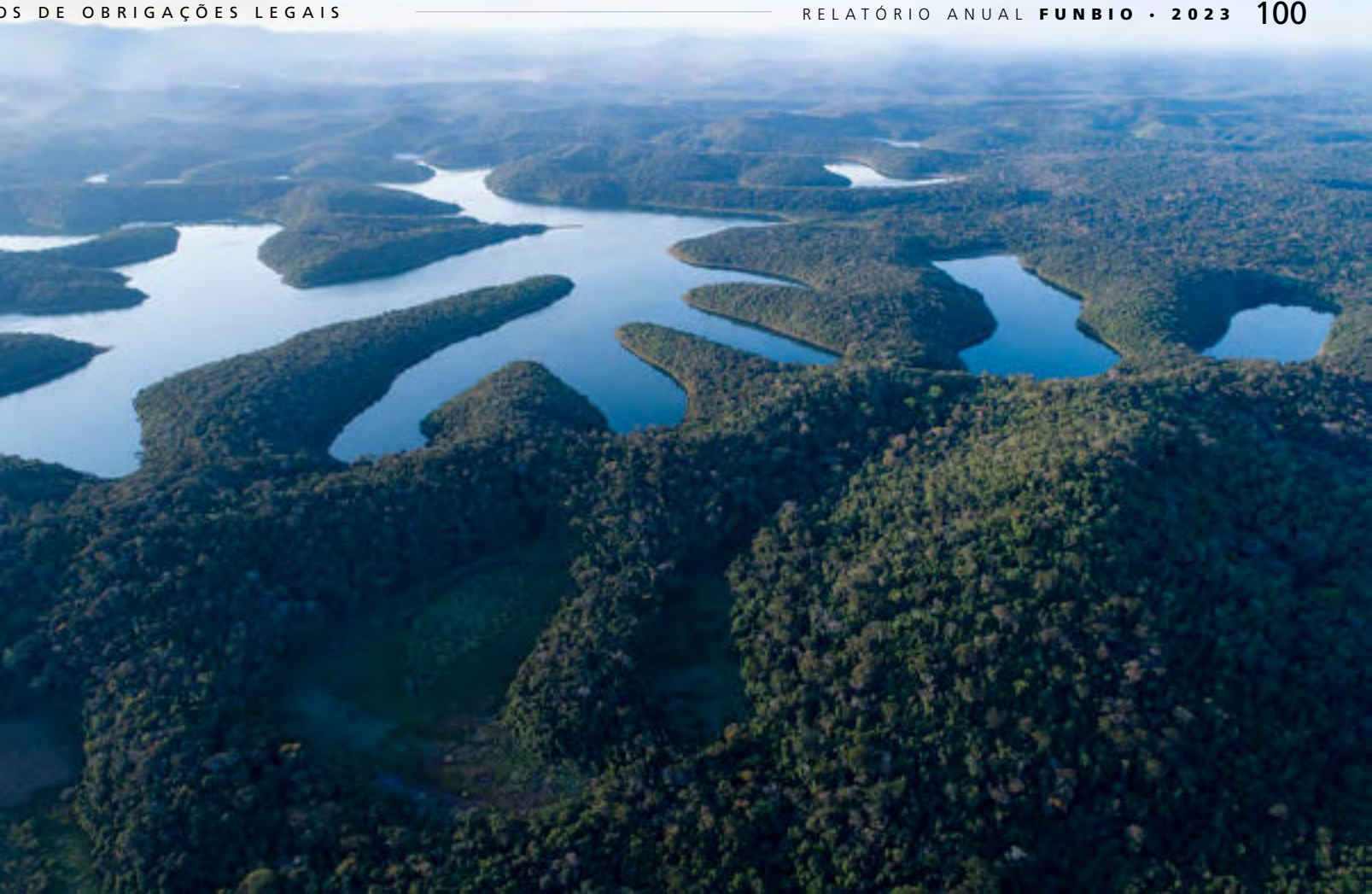
Vista aérea do Parque Estadual do Rio Doce (MG)
